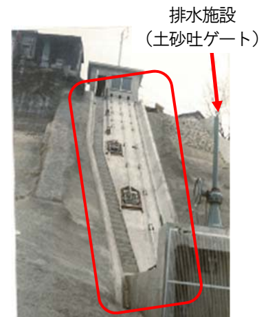
写真3：取水部（斜樋）
